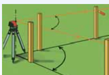
Setzen von rechten Winkeln
